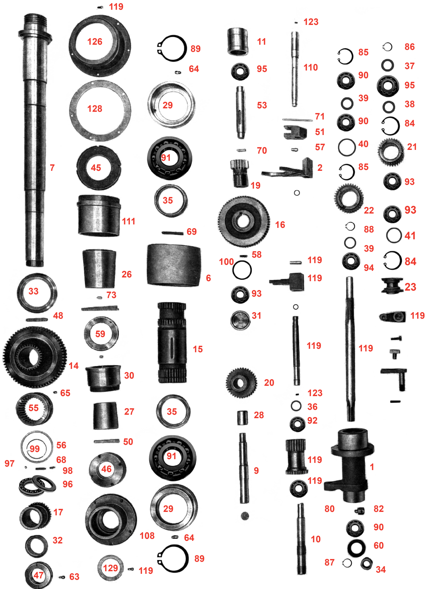
Vreteník 901000
