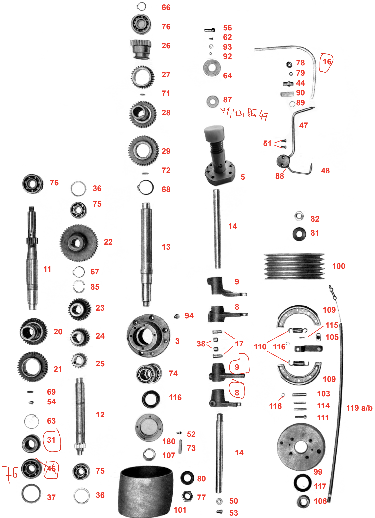
Rýchlostná skriňa 902000
